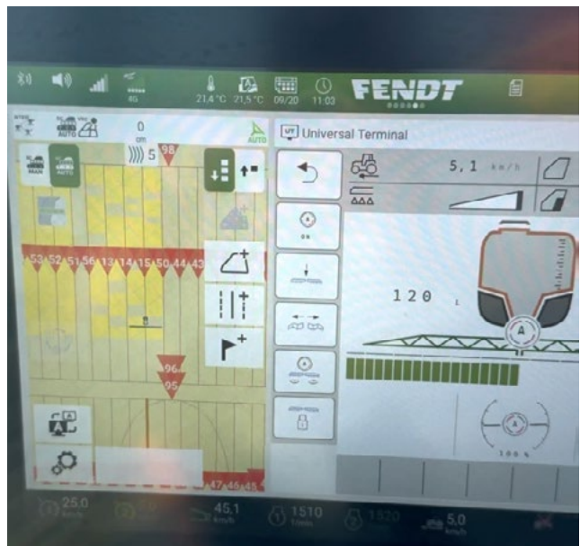
Abbildung 3: Steuerungscomputer auf einer Pflanzenschutzspritze
